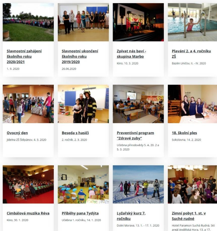
Obr. 4: Podstránka – fotogalerie
